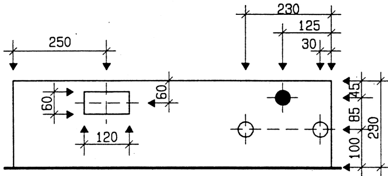
Ansicht oben
