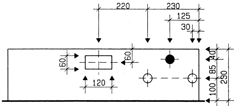
Ansicht oben
