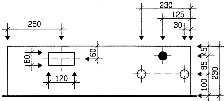
Ansicht oben
