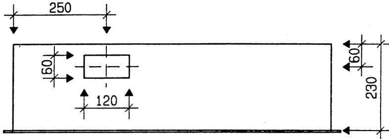
Ansicht oben
