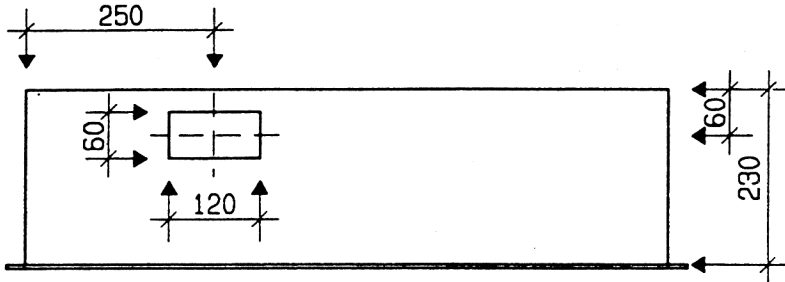
Ansicht oben
