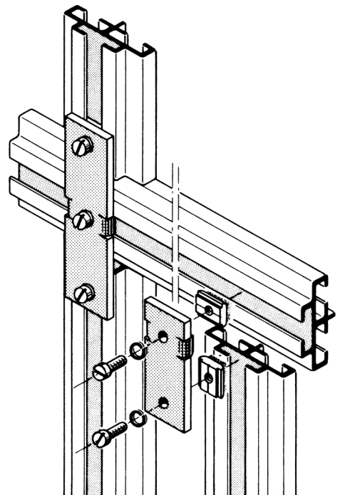
Verbindungsprofile, 3 und 4 Abzweigungen
